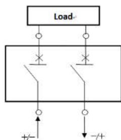
二极串 接线图
