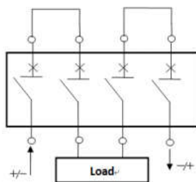
四极串 接线图
