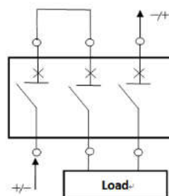
三极串 接线图
